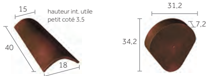
Fronton de rive à rabat pour faîtière demi-ronde
