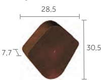
Fronton de rive à rabat pour faîtière bout-à-bout angulaire
