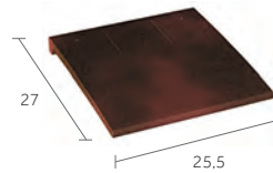
Tuile et demie
